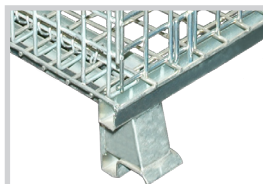
Stapellaschen im Standfuß integriert um mehrere Palettencon- tainer sicher stapeln zu können.
