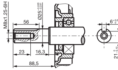
MOTORWELLE KW25x88,5 (S2)
