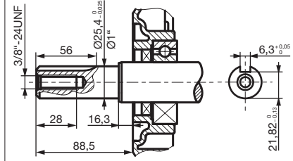
MOTORWELLE KW1“(25,4)x88,5 (Q1)
