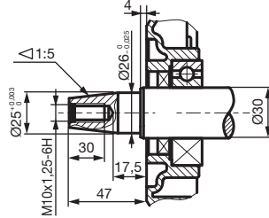
MOTORWELLE TP26x47 (V3)
