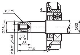
MOTORWELLE TP26x77,5 (V2)
