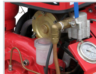
Integrierte Vorförderpumpe Über die Flügelzellenvorförderpumpe kann der Saugtrakt mit Wasser befüllt werden. Ein zeitraubendes Vorfüllen entfällt.
