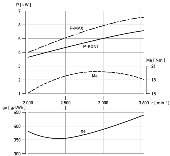
EG4-0420 P: Leistungskurve, Me: Drehmomentkurve, ge: Verbrauchskurve
