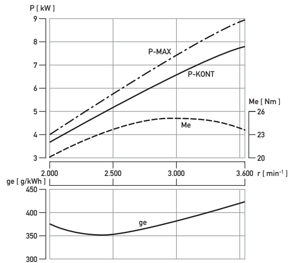
EG4-0390 P: Leistungskurve, Me: Drehmomentkurve, ge: Verbrauchskurve
