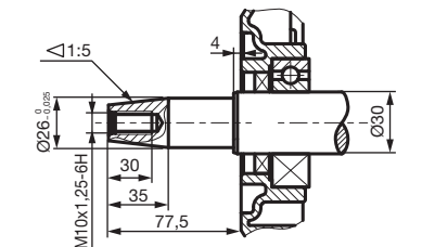
MOTORWELLE TP26x77,5 (V2)
