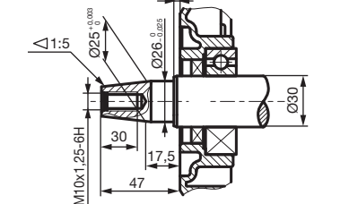
MOTORWELLE TP26x47 (V3)
