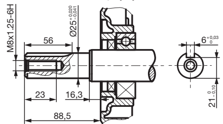
MOTORWELLE KW25x88,5 (S2)
