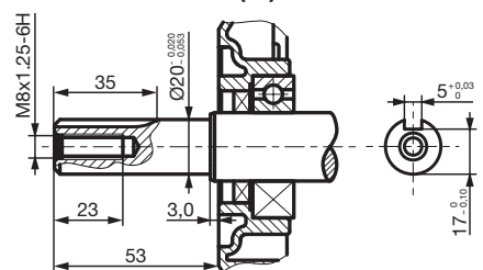
MOTORWELLE KW20x53 (S1)
