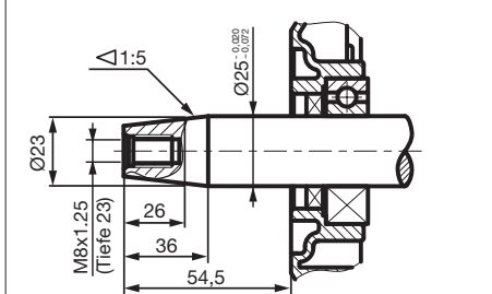
MOTORWELLE TP25x54,5 (V5)
