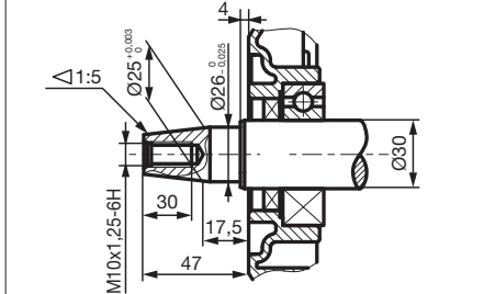
MOTORWELLE TP26x47 (V3)
