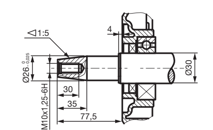
MOTORWELLE TP26x77,5 (V2)
