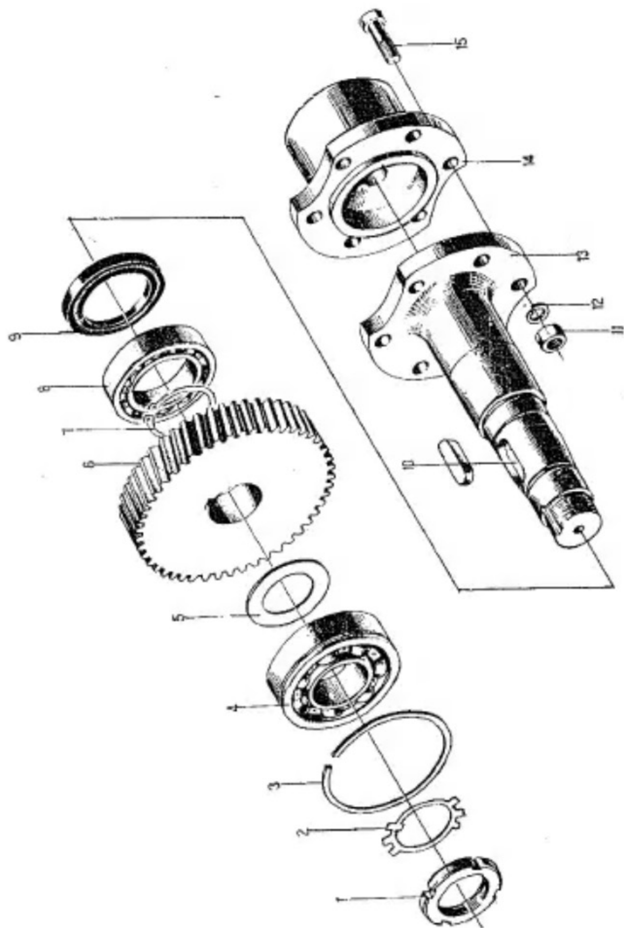
输出轴部件 Output Shaft Assembly
