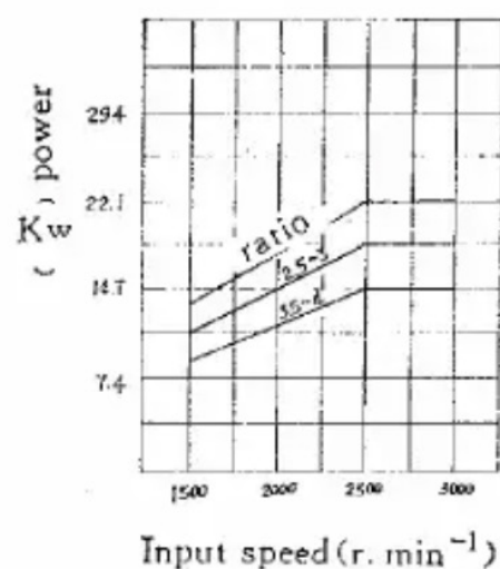
MA100 齿轮箱
