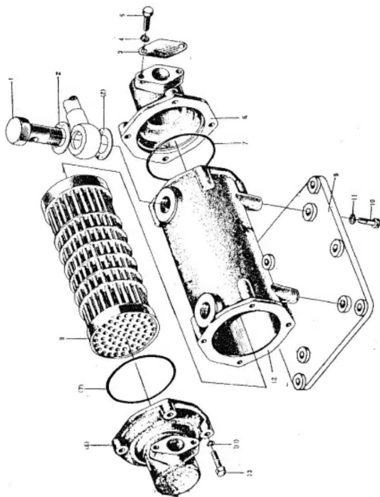
冷却器部件 Cooler Assembly
