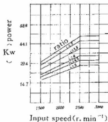
MA125 齿轮箱
