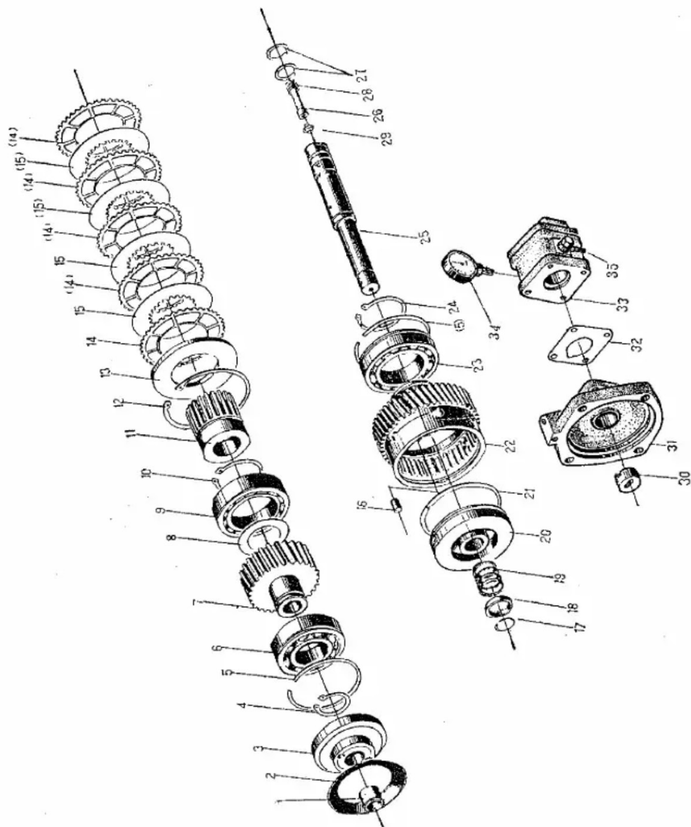
传动轴部件 Transmission Shaft Assembly
