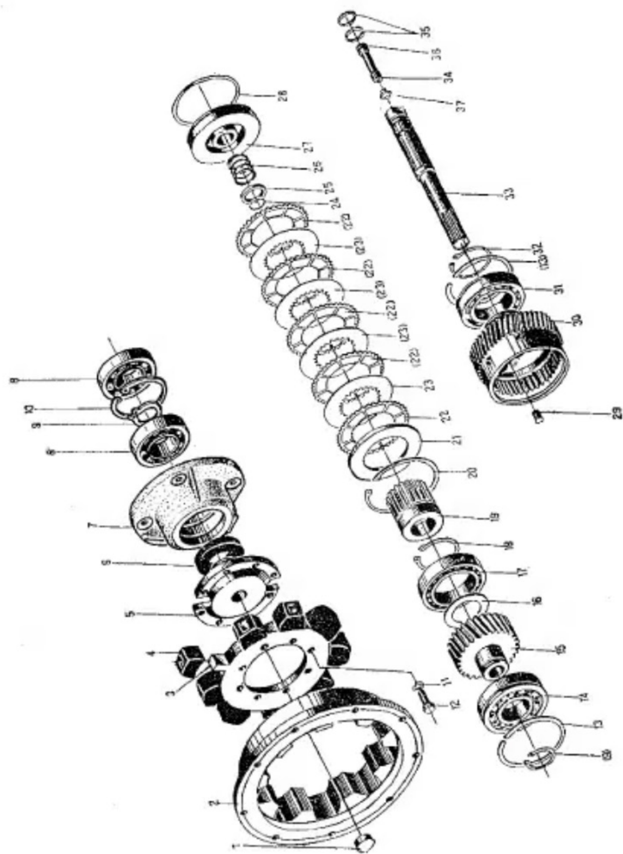
输入联轴节、输入轴零件 Input Coupling, Input Shaft Assembly
