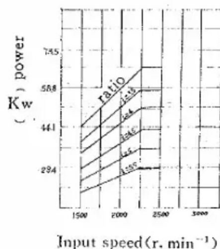
MA142 齿轮箱
