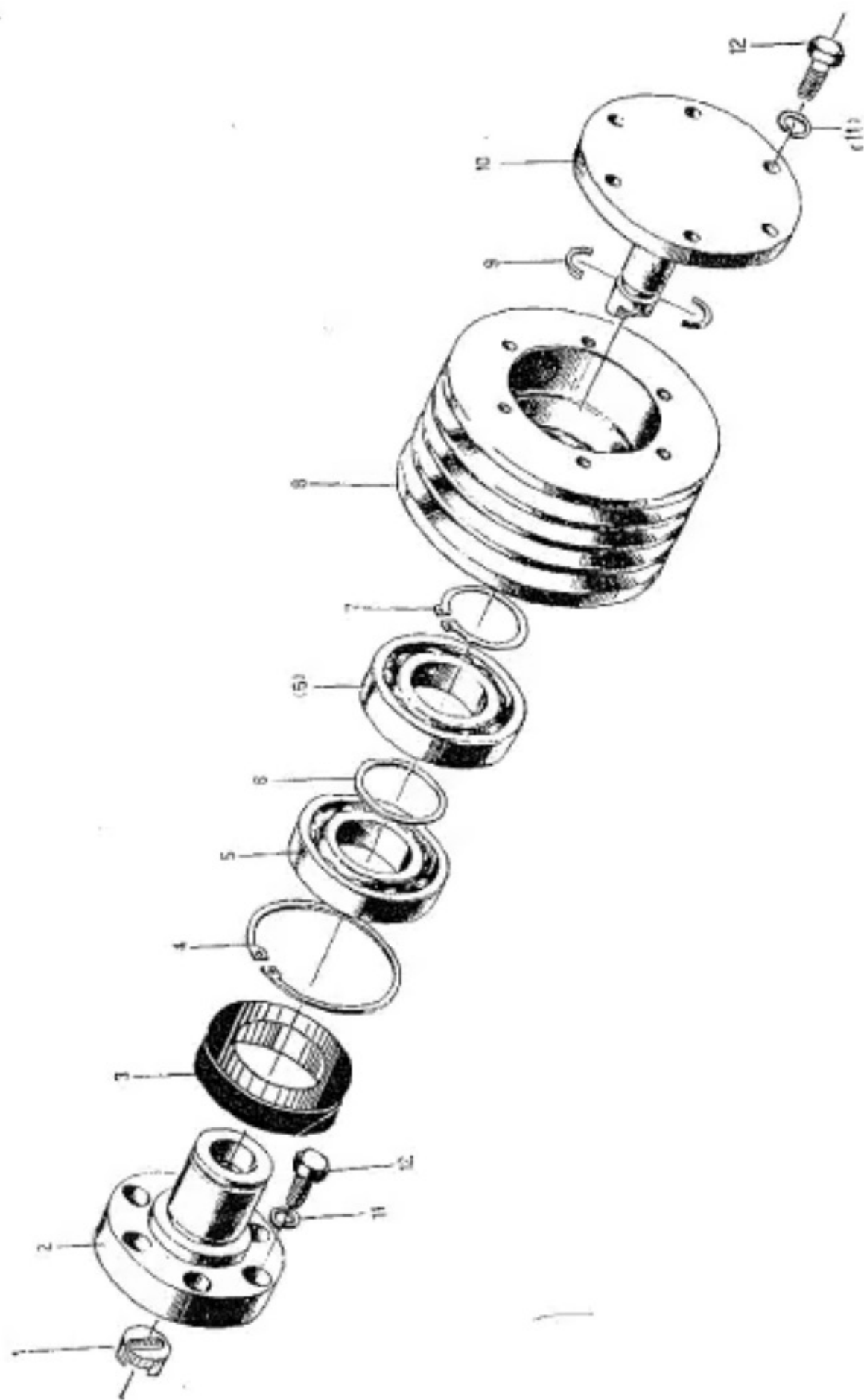
MA 125A 齒輪箱輔助功率輸出軸部分 MA 142A MA125A, MA142A P. T. O Assembly
